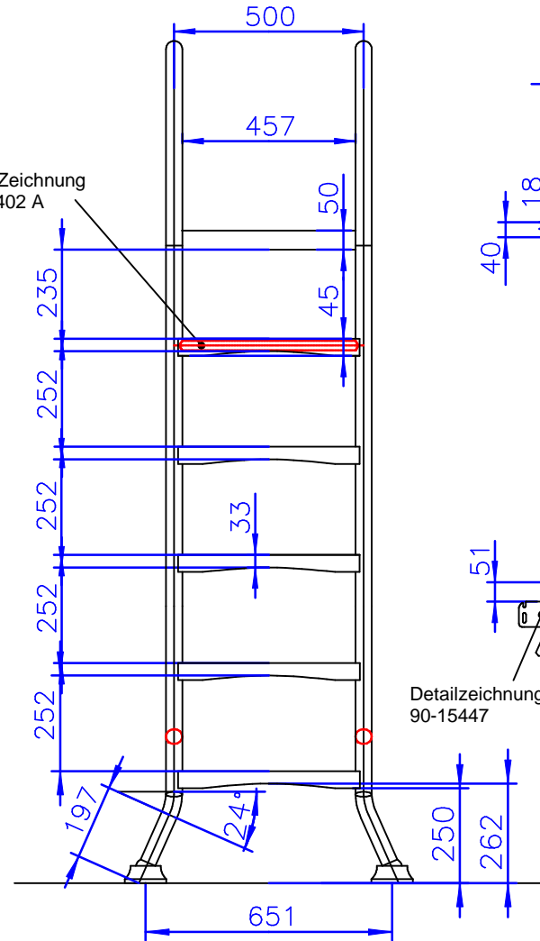
Ansicht "A"
